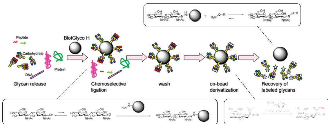
図1 グライコブロットング法の原理と基本的なプロトコル
